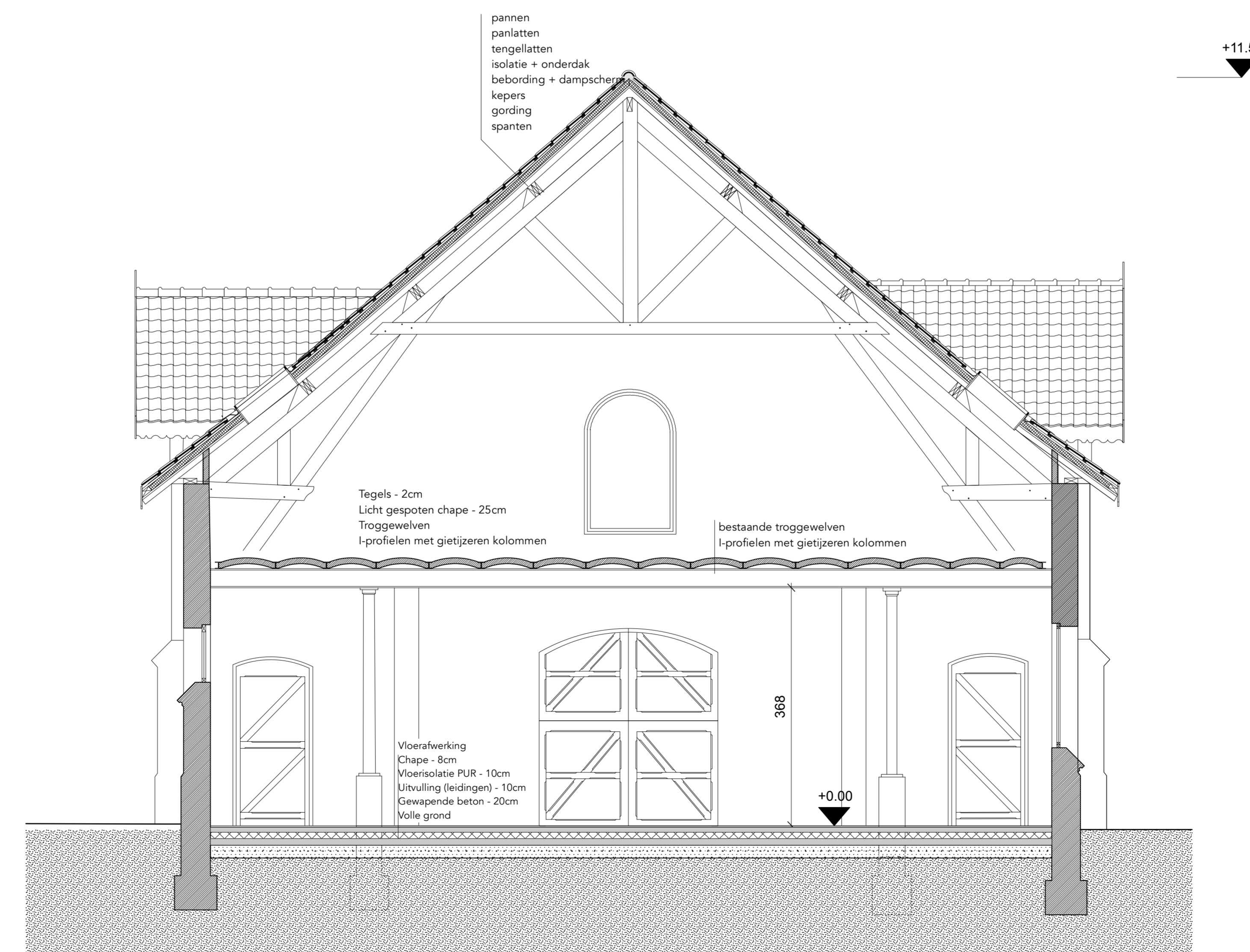
SNEDE D-D'
