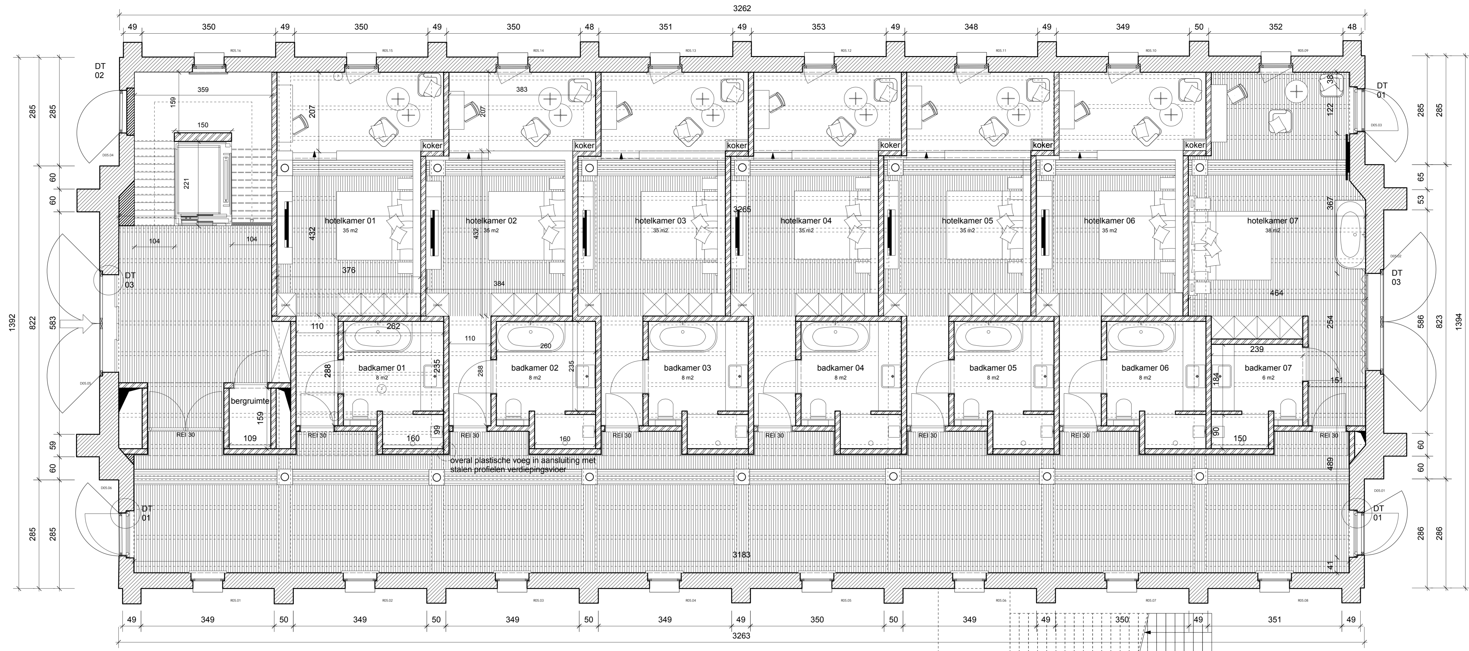
Grondplan Schaal: 1:50
