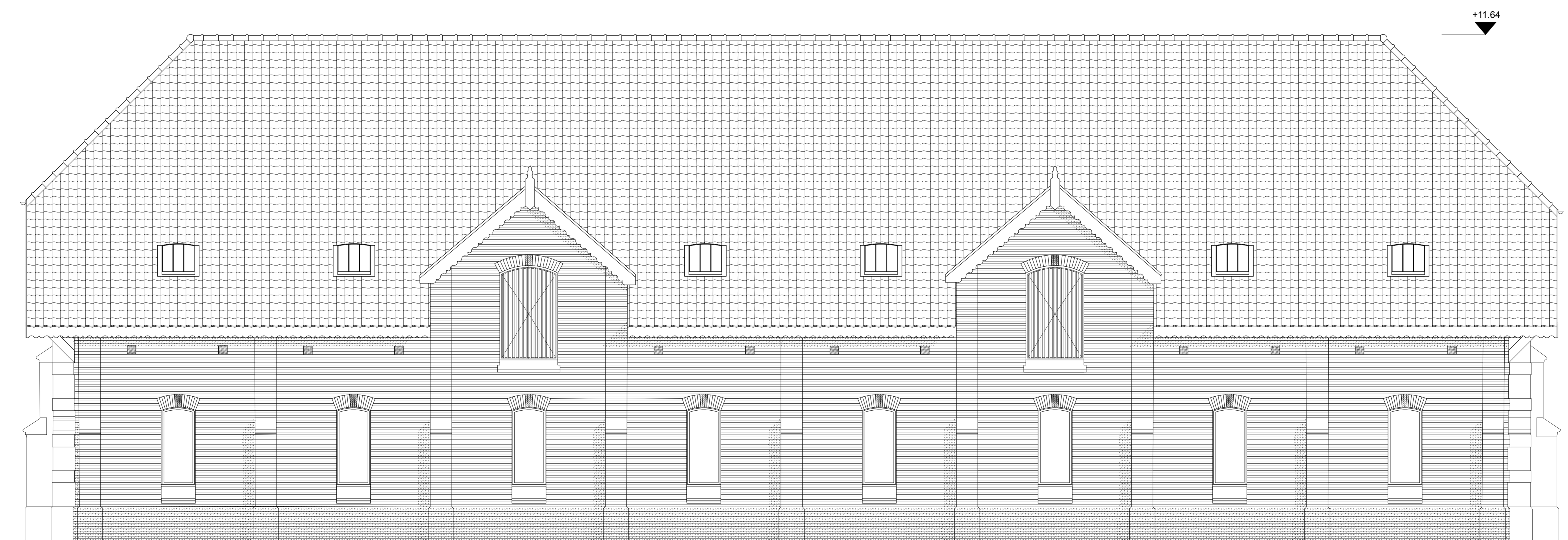
Westelijke gevel
