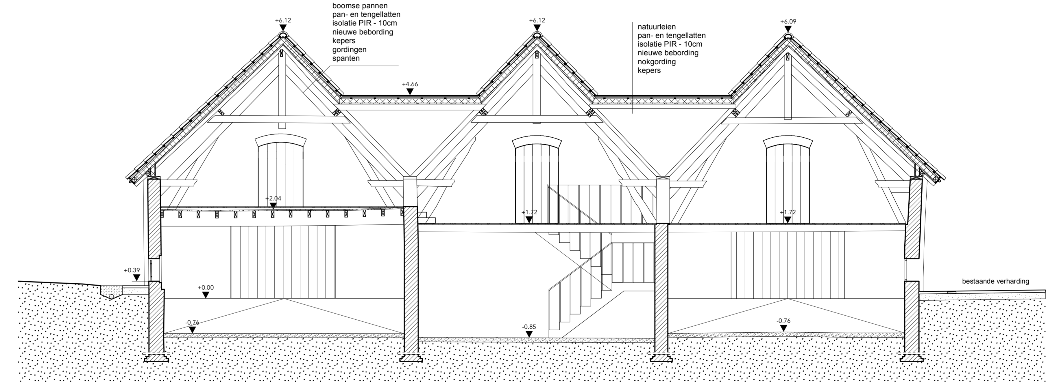
SNEDE EE'
