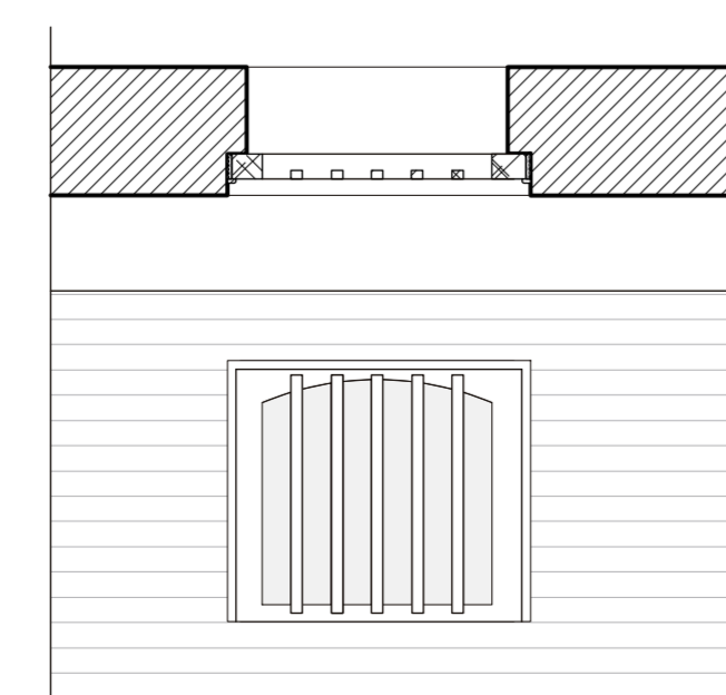
detail binnenraam - schaal 1/20
