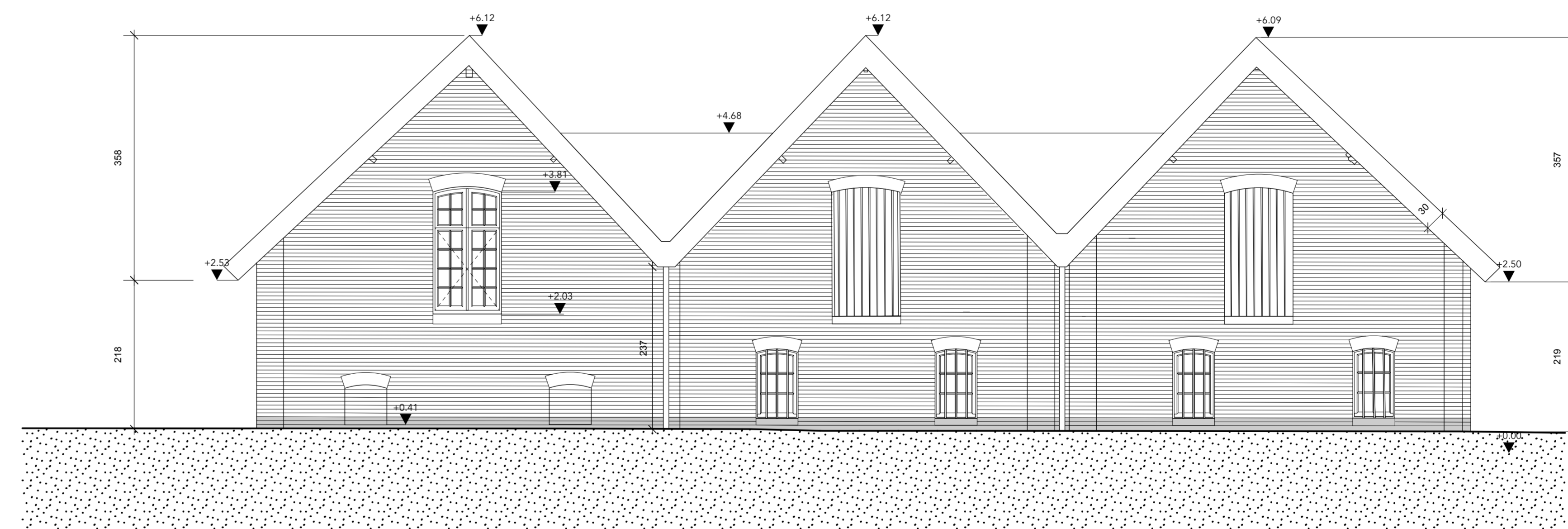
WESTGEVEL
