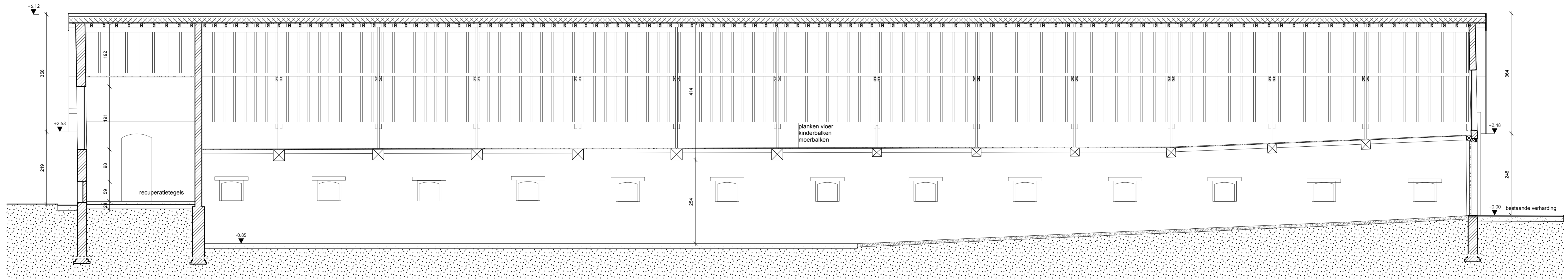
DOORSNEDE A-A'
