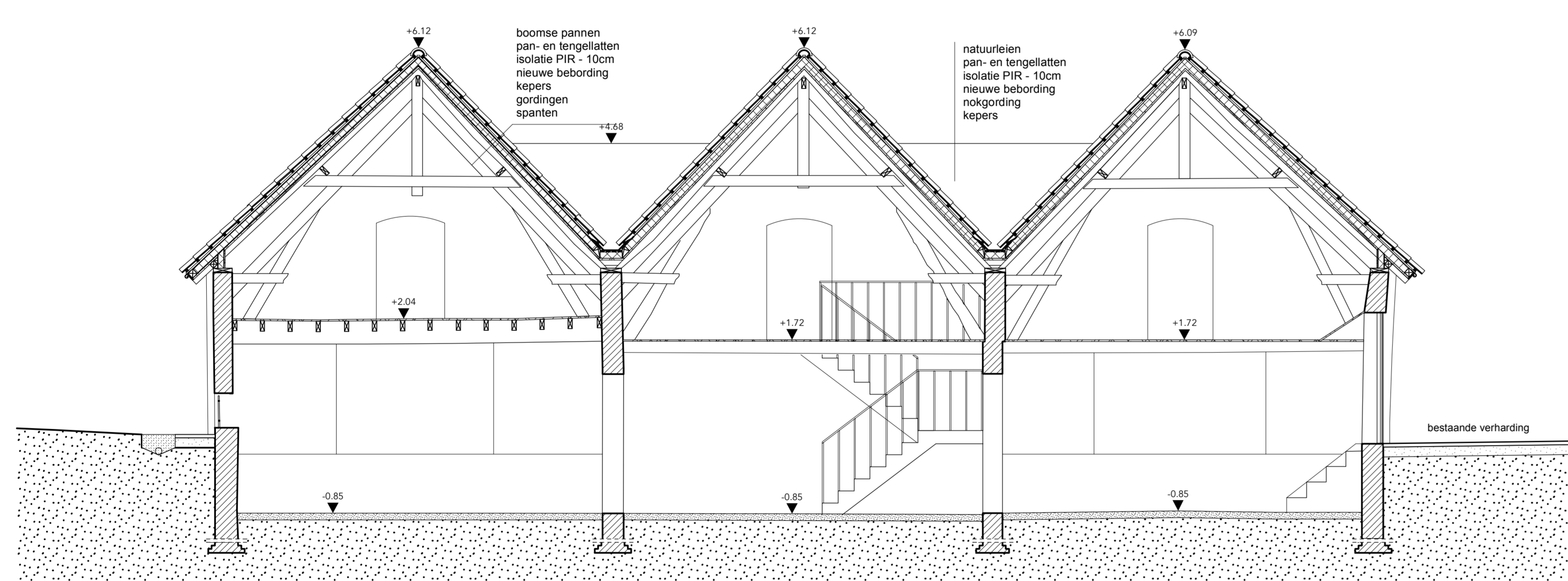
SNEDE DD'
