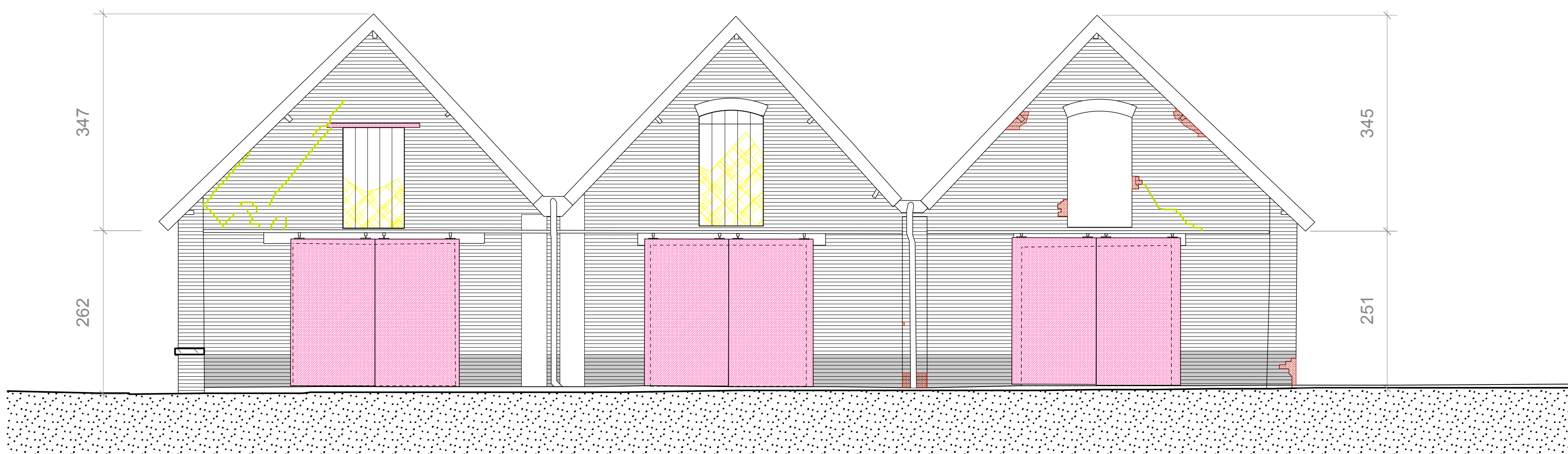
OOSTGEVEL
