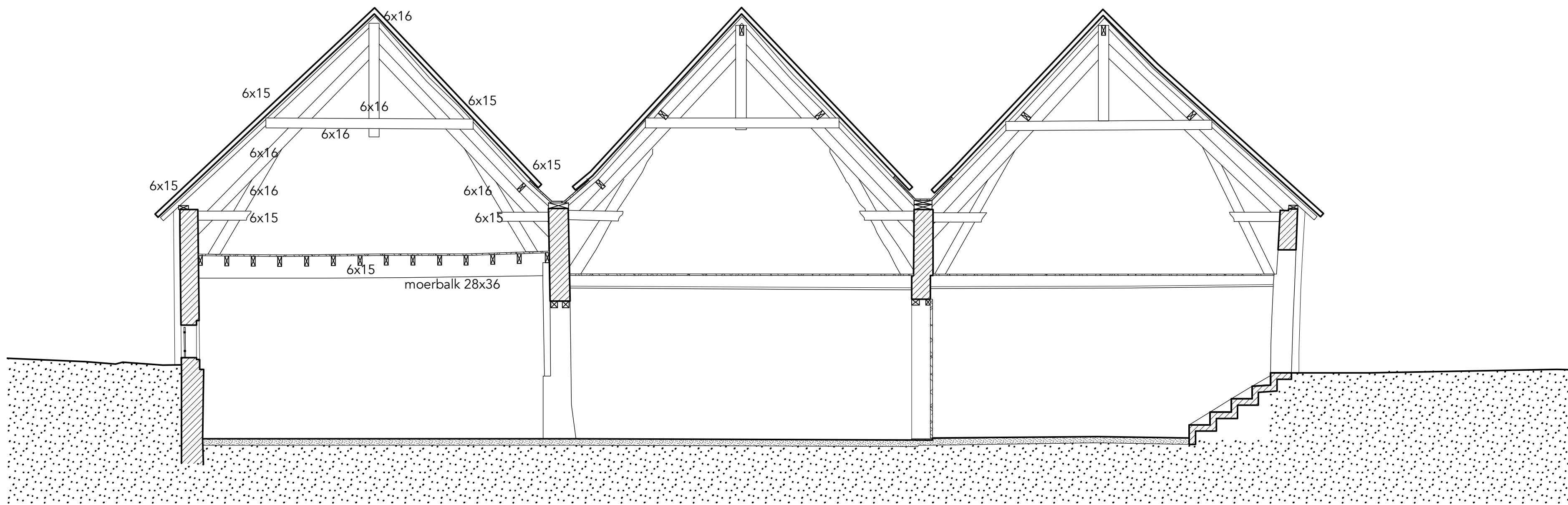
SNEDE BB'
