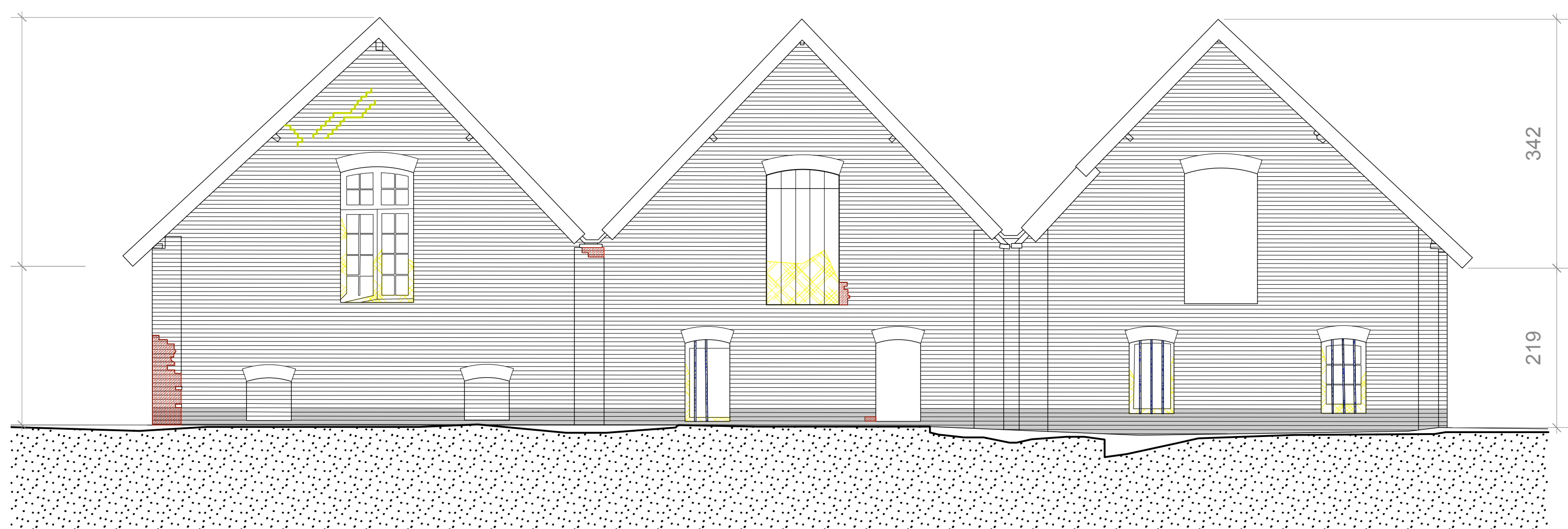
WESTGEVEL
