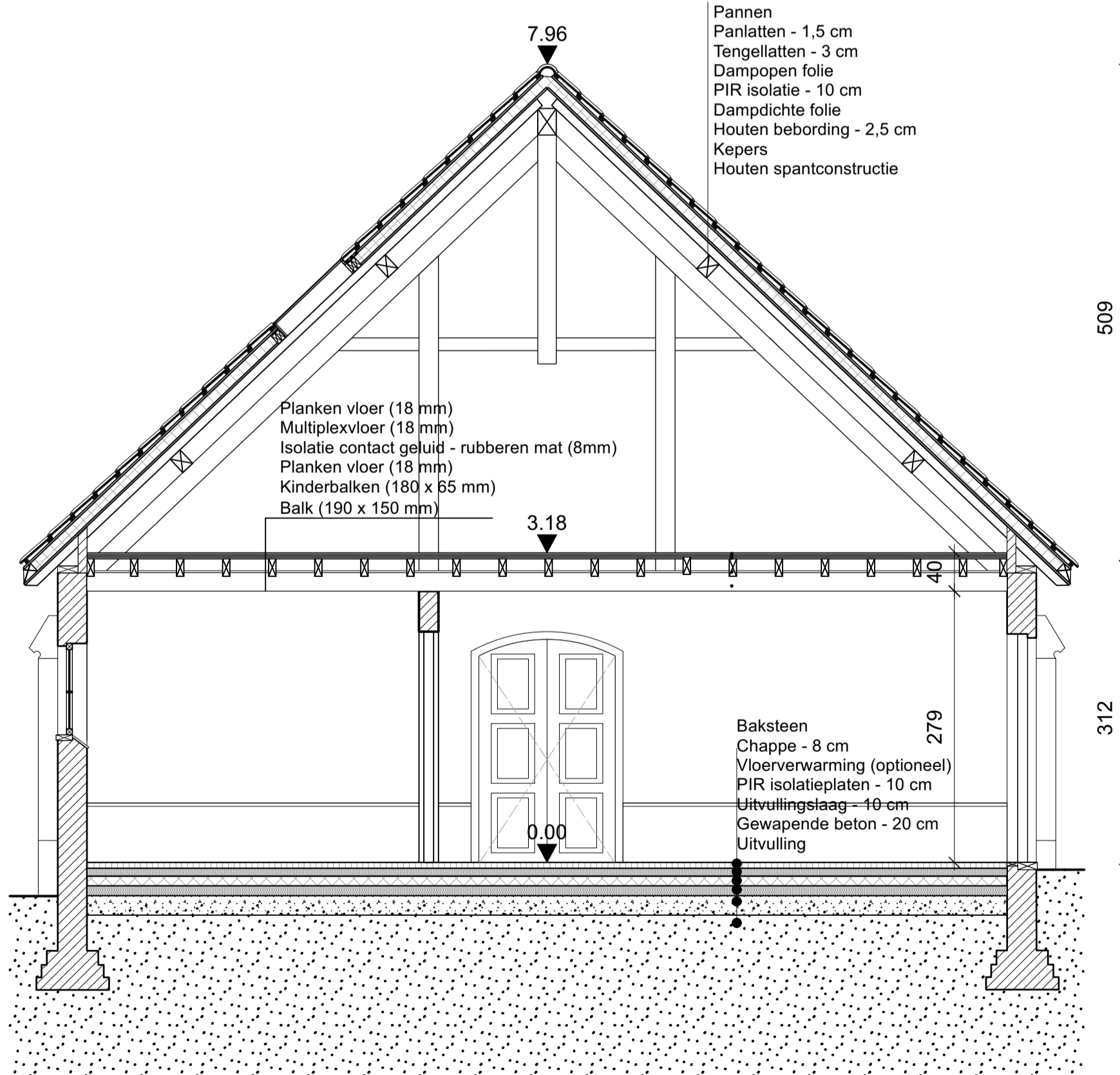
DOORSNEDE D 1/50
