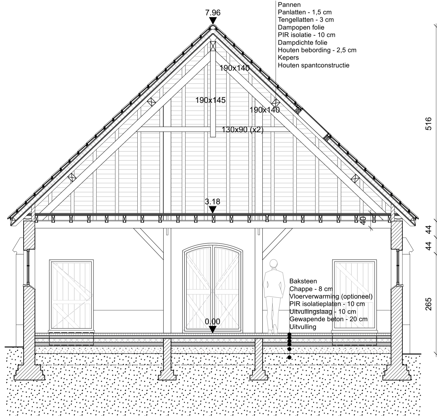
DOORSNEDE B 1/50
