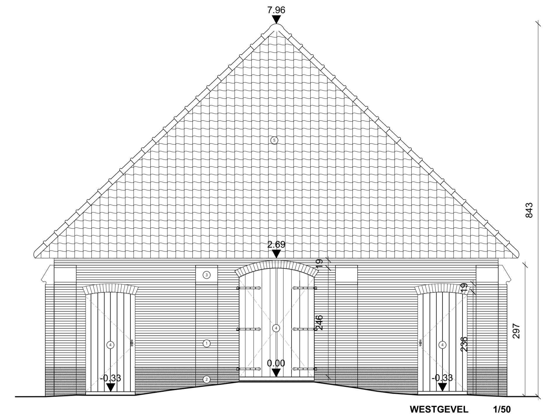
WESTGEVEL 1/50
