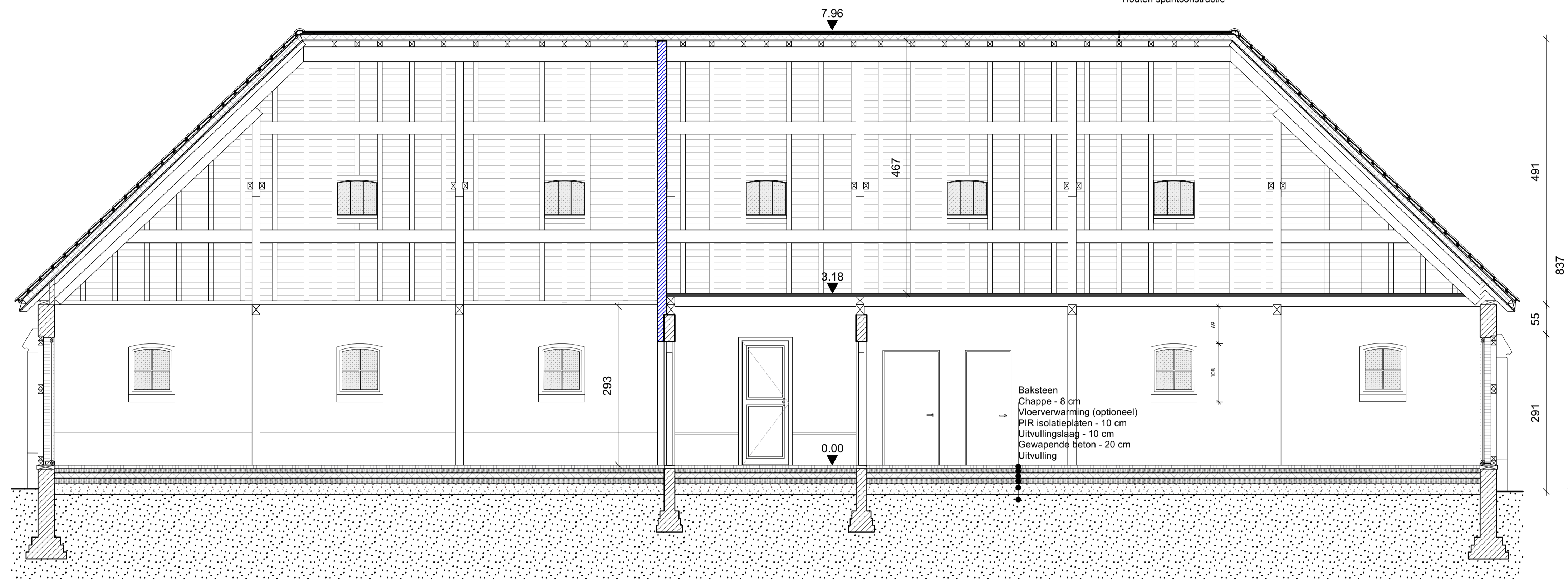
DOORSNEDE A 1/50
