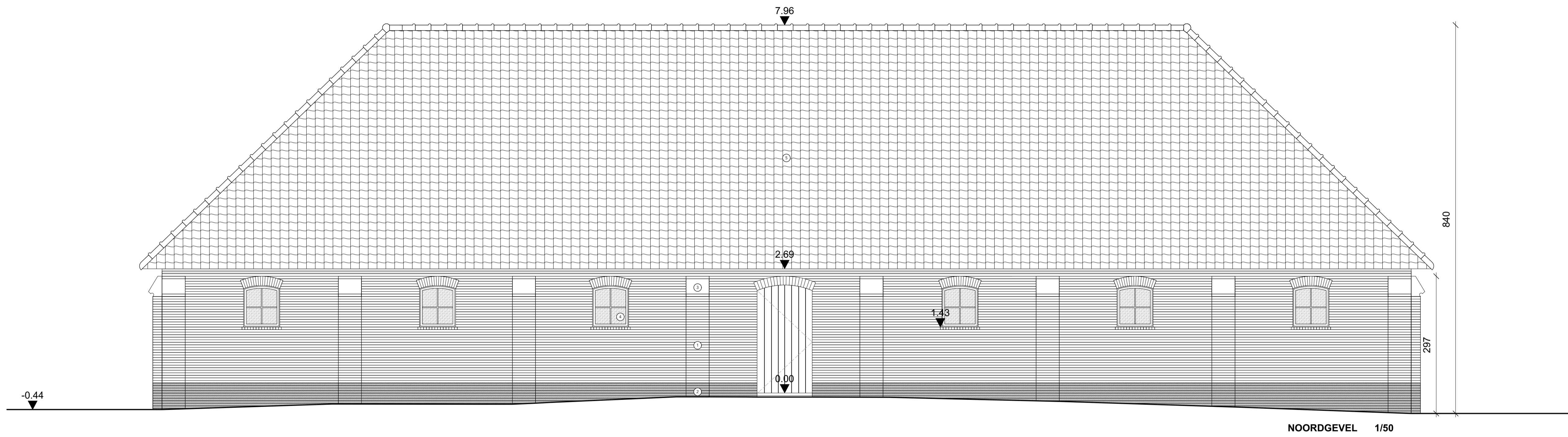
NOORDGEVEL 1/50
