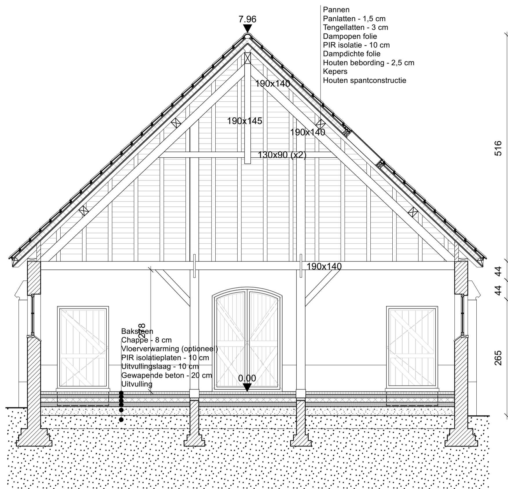
DOORSNEDE C 1/50
